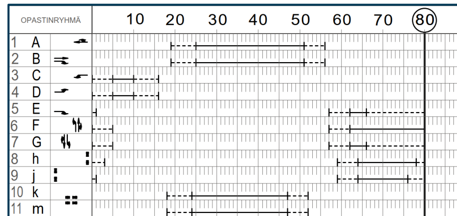
Kuva 6. Aamuhuipputunti - ajoituskaavio
