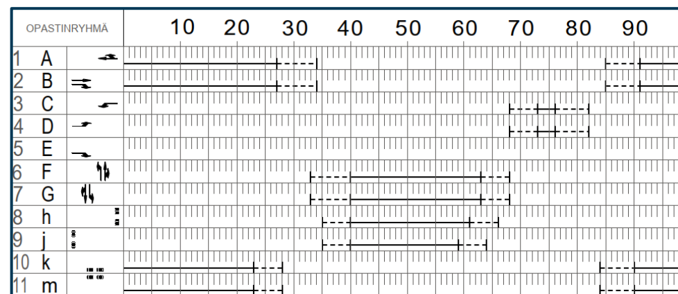
Kuva 7. Iltahuipputunti - ajoituskaavio
