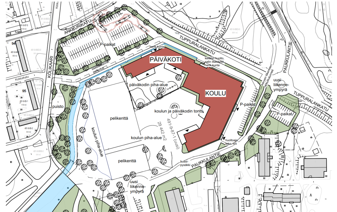
Kuva 20. Hankesuunnitelma
